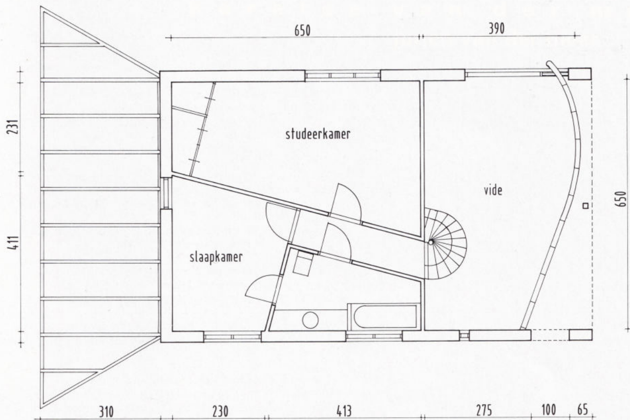
verdieping
