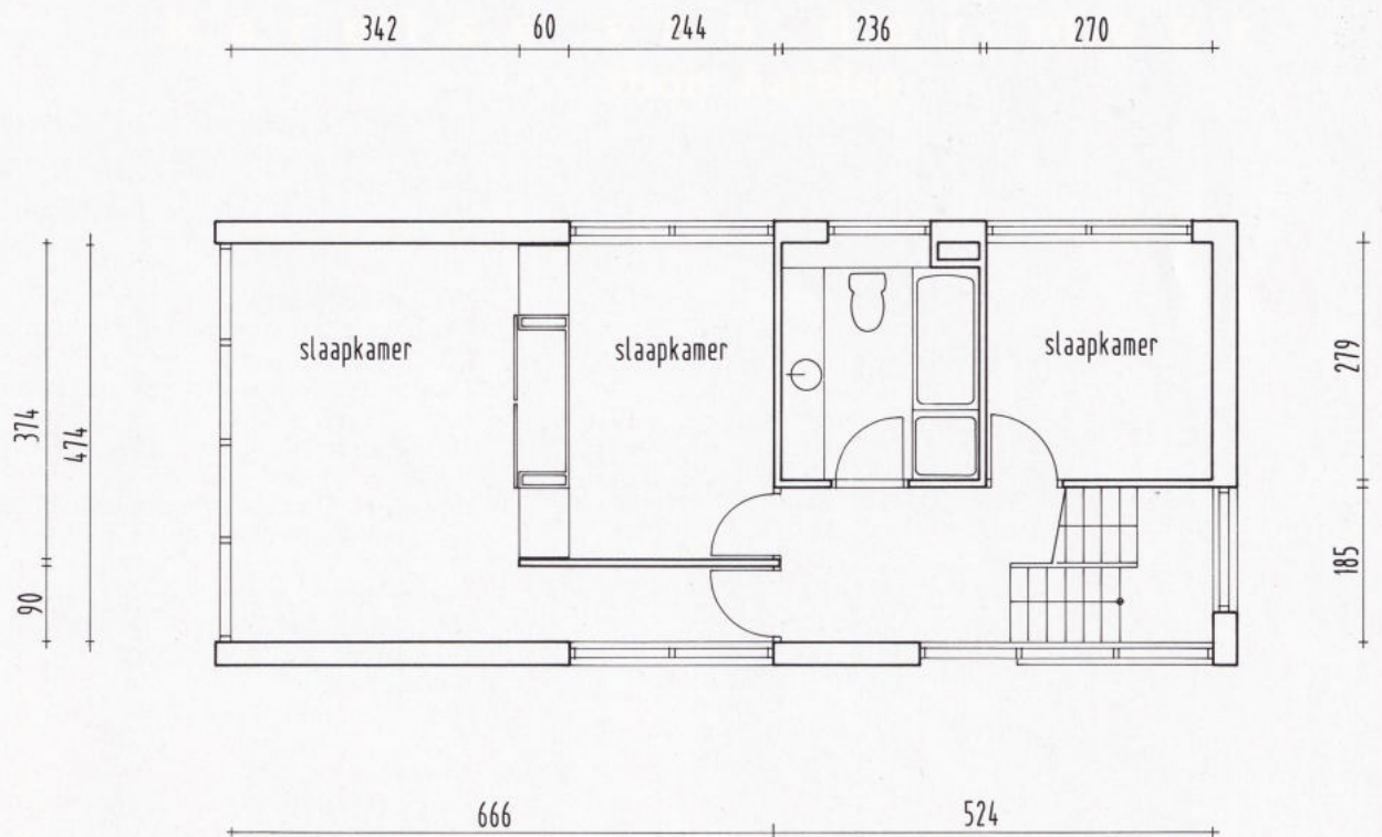
verdieping
