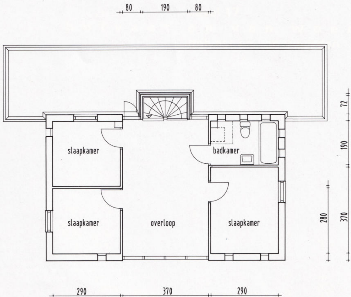
verdieping
