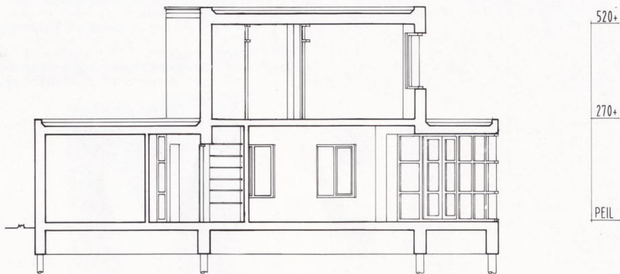
langsdoorsnede
