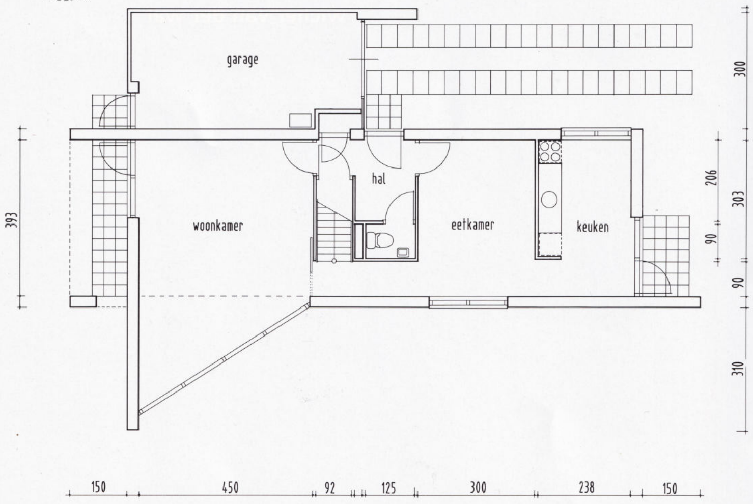
schaal 1:100
