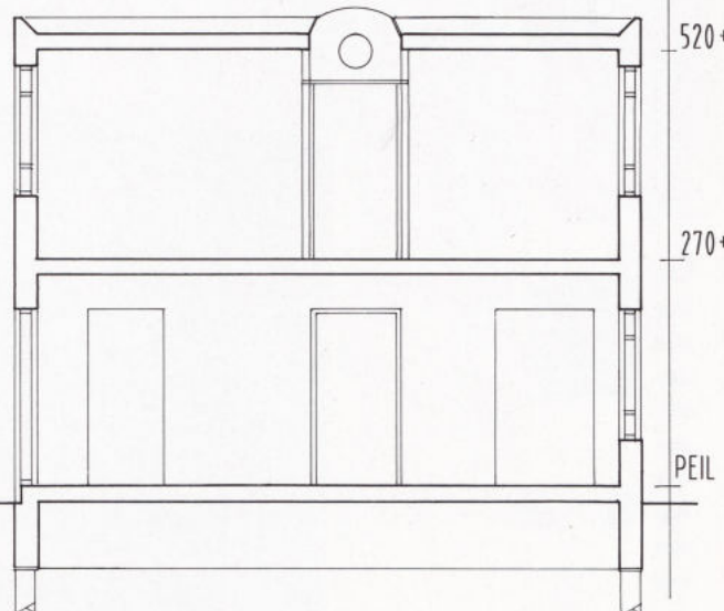
doorsnede b
