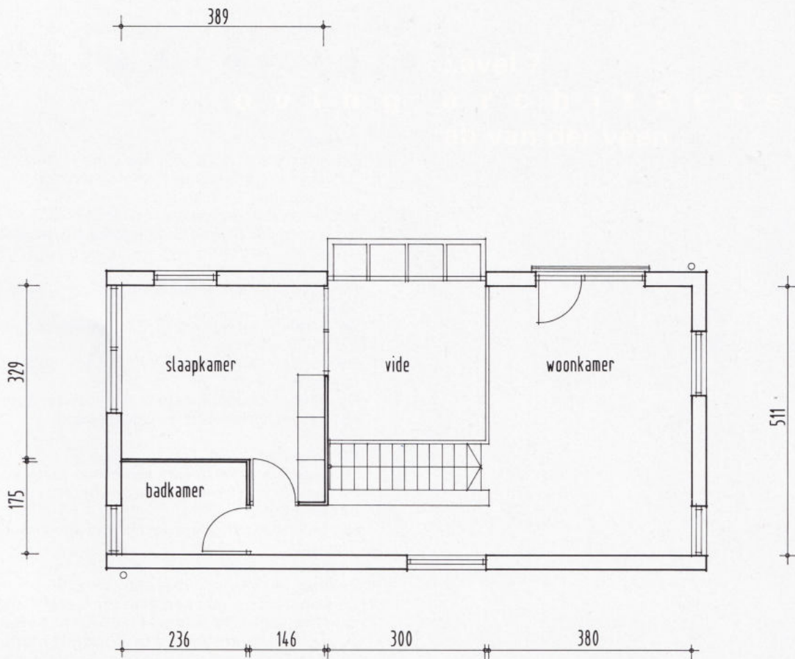
verdieping
