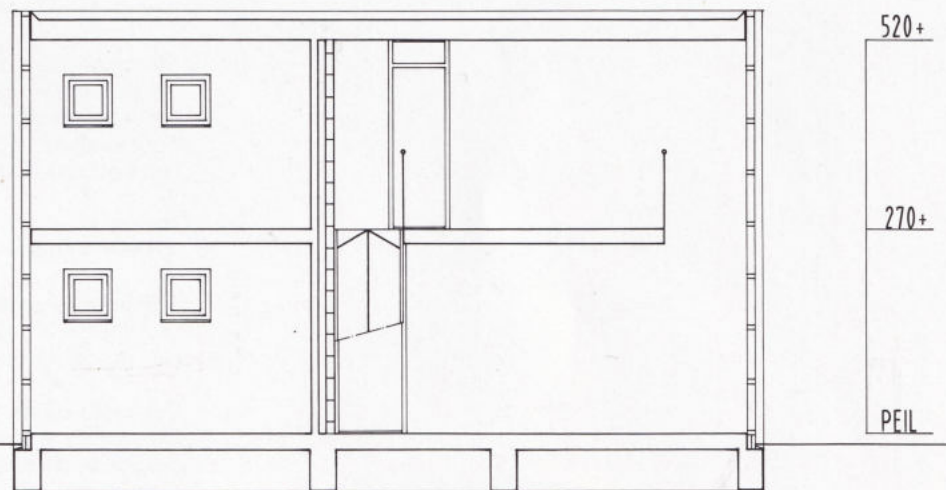
langsdoorsnede
