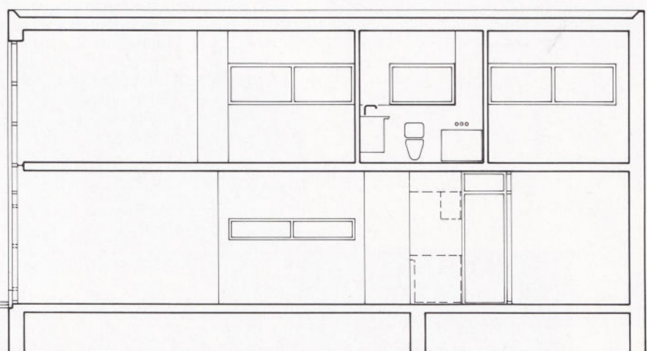
doorsnede
