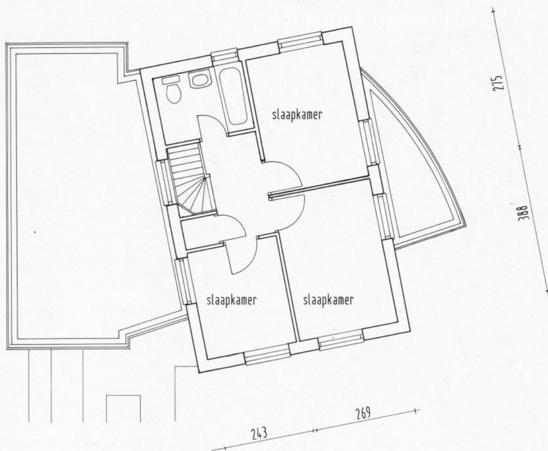
verdieping
