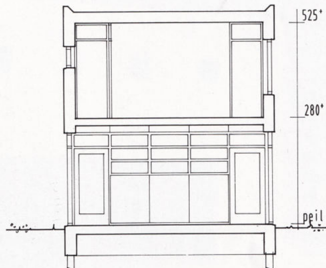
dwarsdoorsnede
