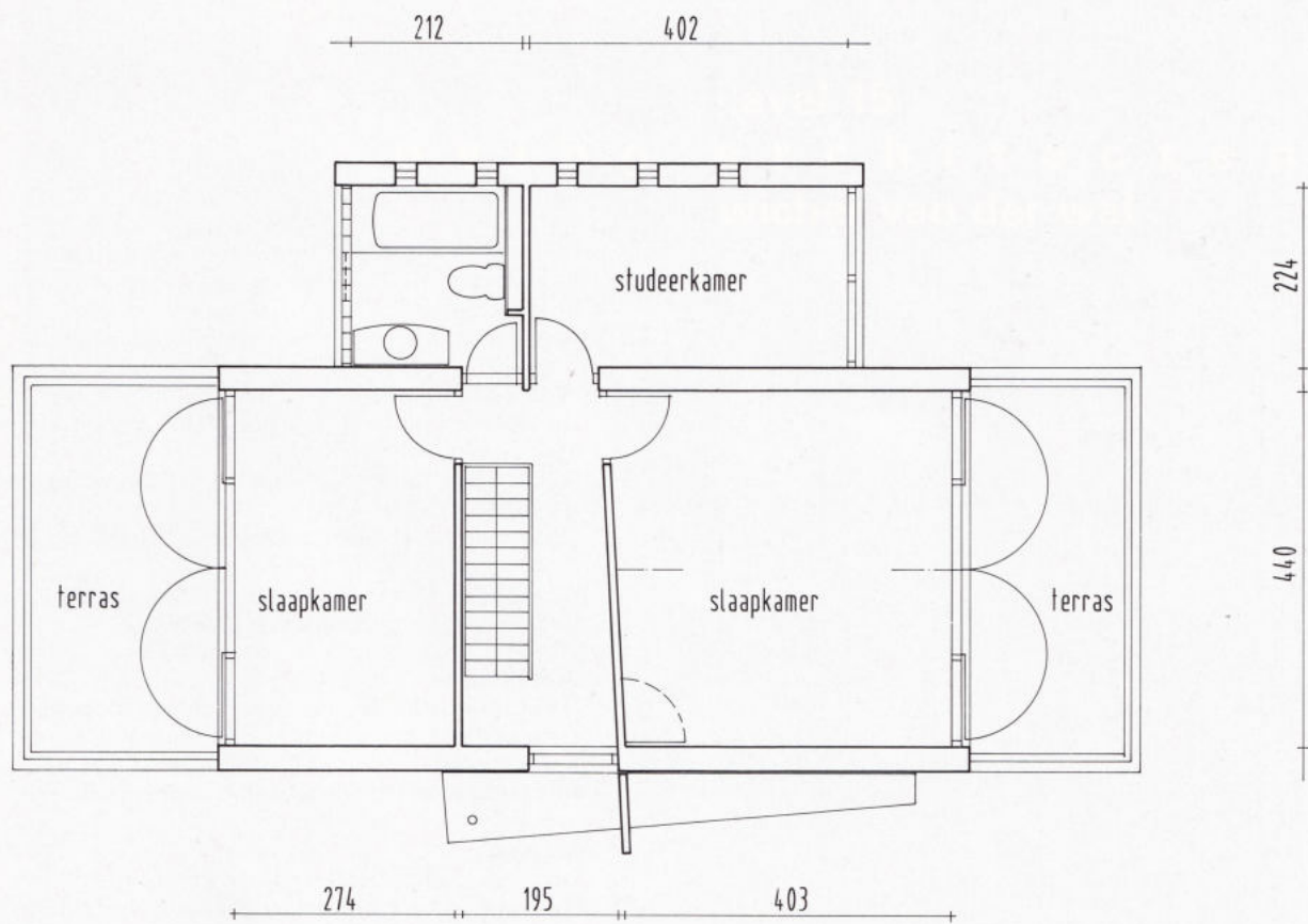
verdieping
