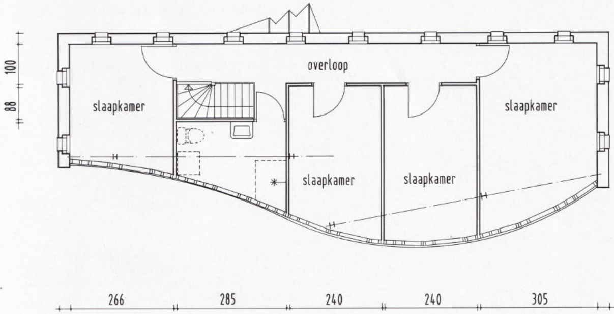
verdieping
