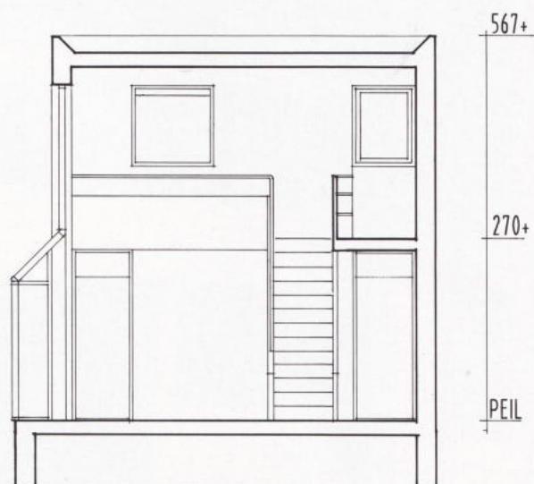
doorsnede
