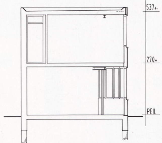
dwarsdoorsnede
