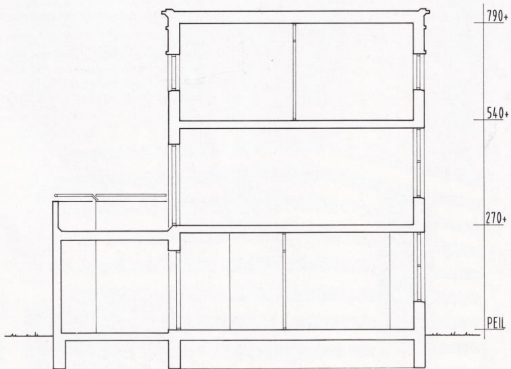
langs-doorsnede
