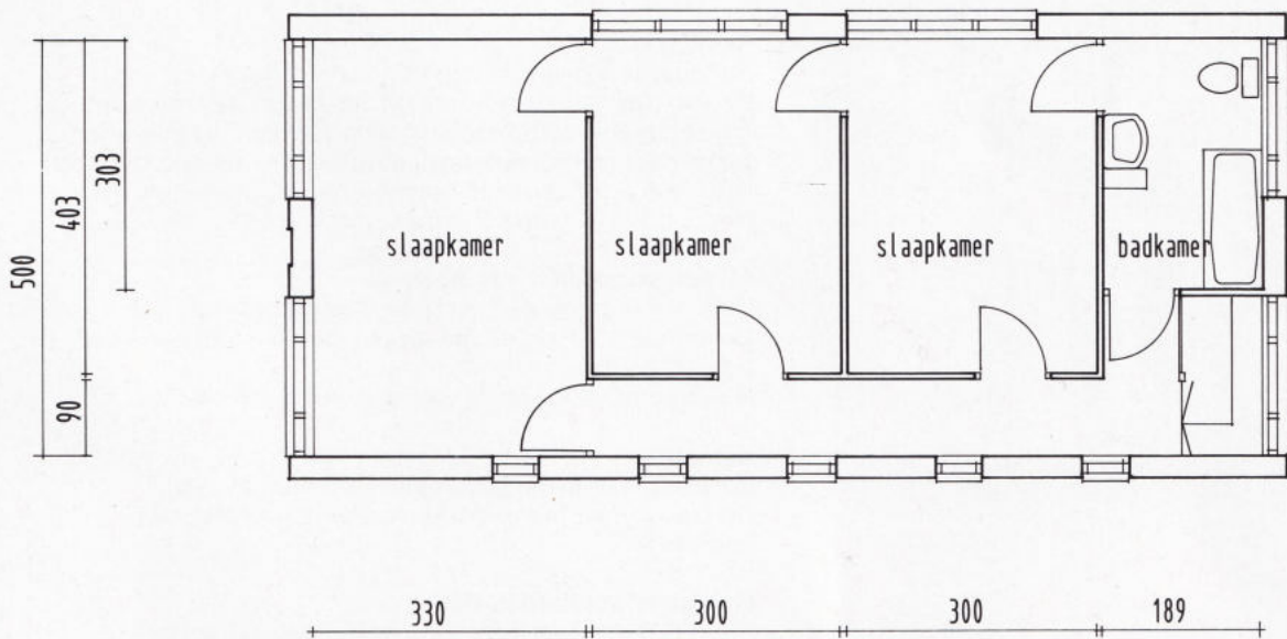
verdieping
