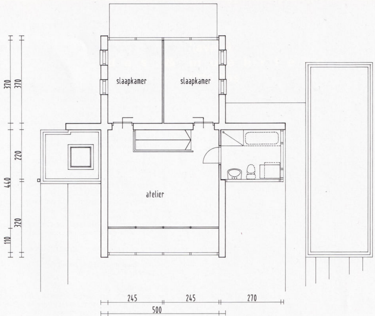
verdieping
