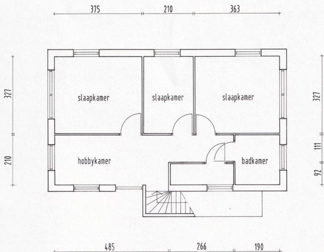
verdieping
