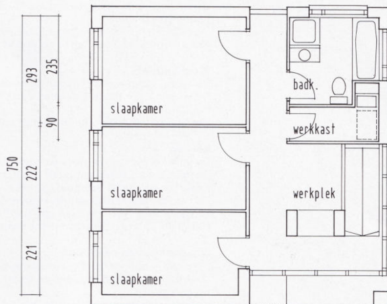
verdieping
