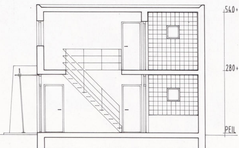
doorsnede
