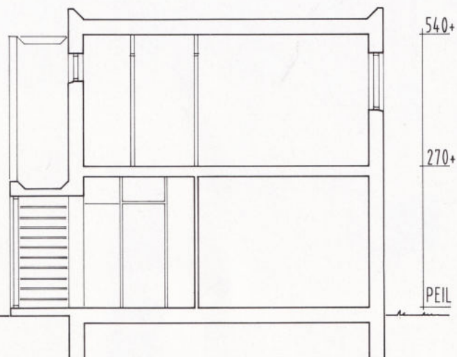
doorsnede
