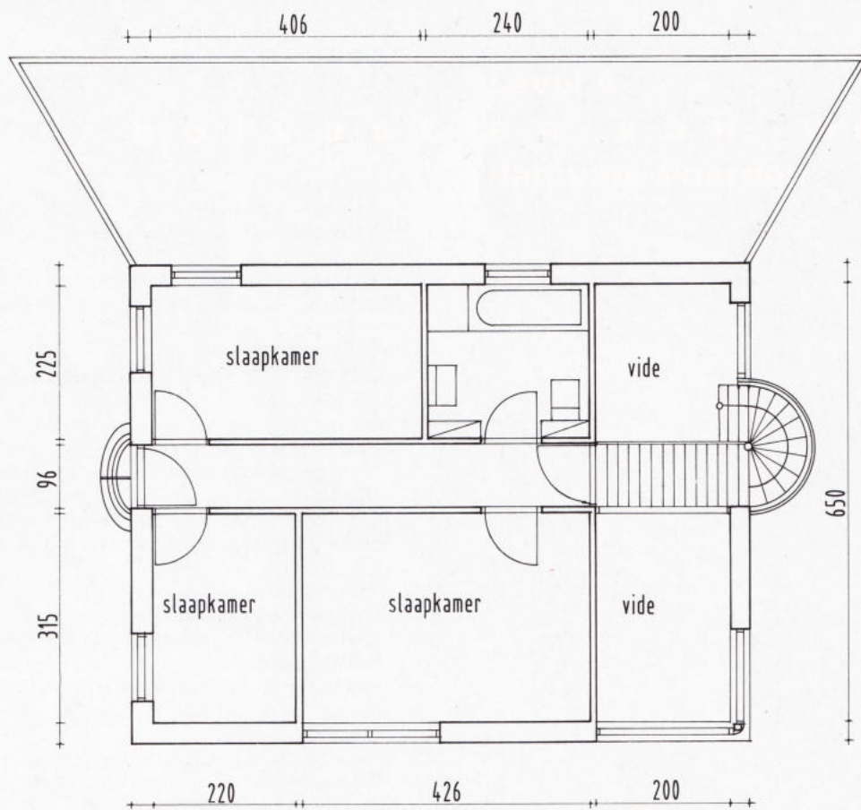
verdieping
