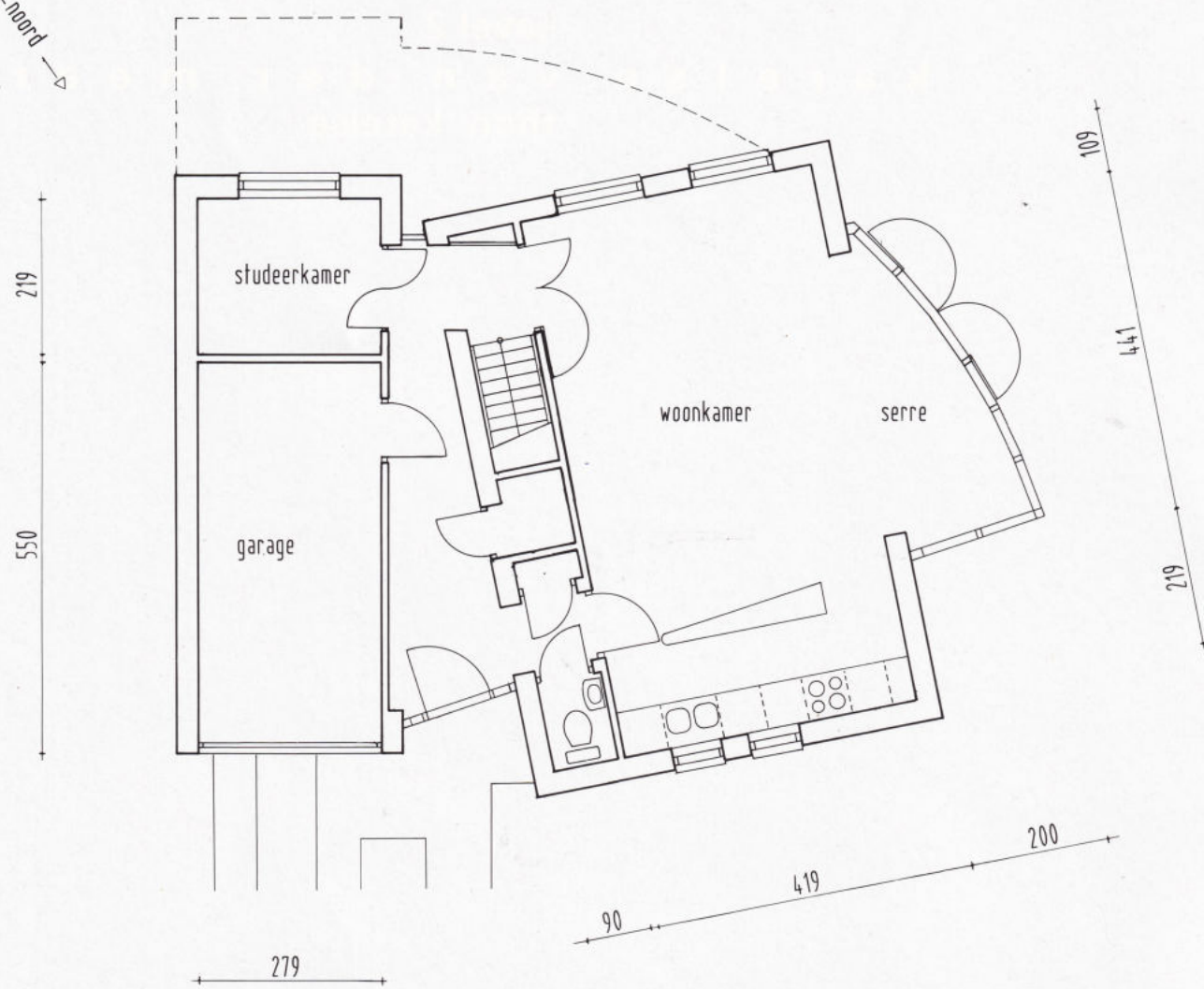
schaal 1:100
