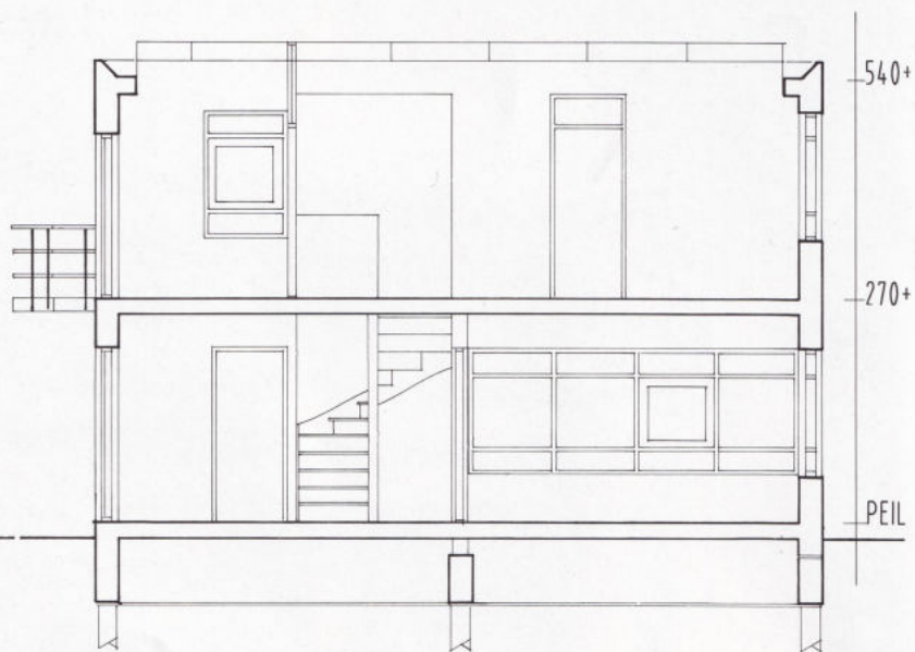
doorsnede
