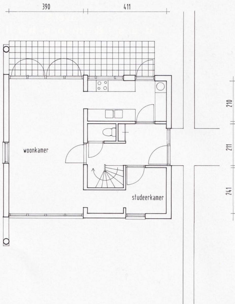
schaal 1:100
