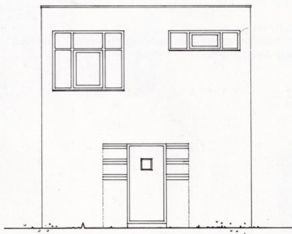
noord-oost gevel
